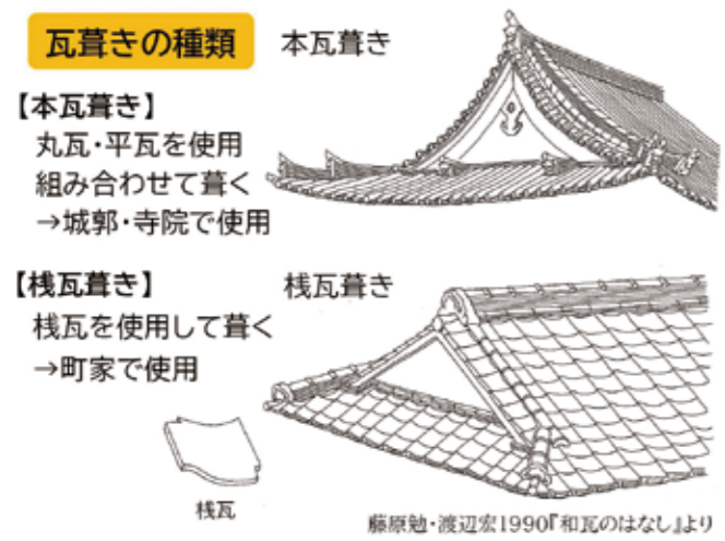
図8 瓦の葺き方
