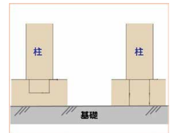
図6 土台
