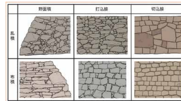
図3 石垣の積み方
