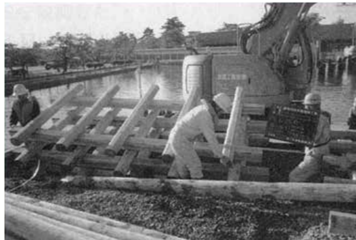
図9-2 梯子胴木
