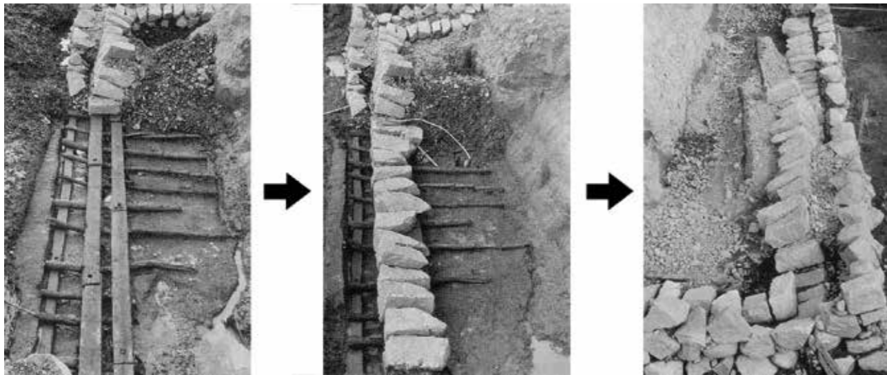
図8 石垣の基礎
